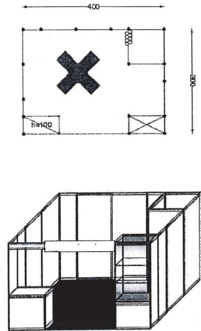
TYPE „A“ STANDARD DESIGN
